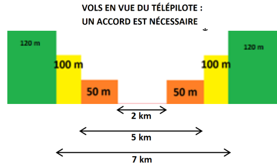
Vue transversale
