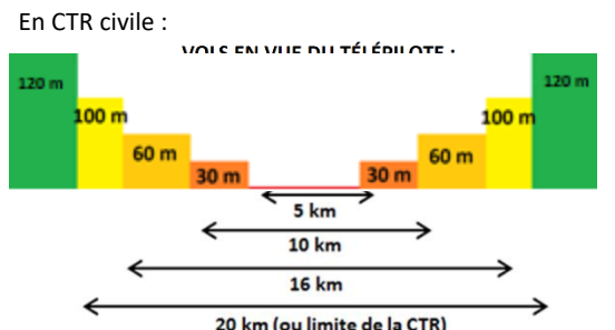
Vues transversales
